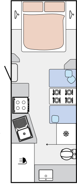
595 BLACKHAWK (ANGLE KITCHEN)
